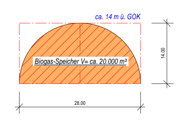
Schnitt Gasspeicher
